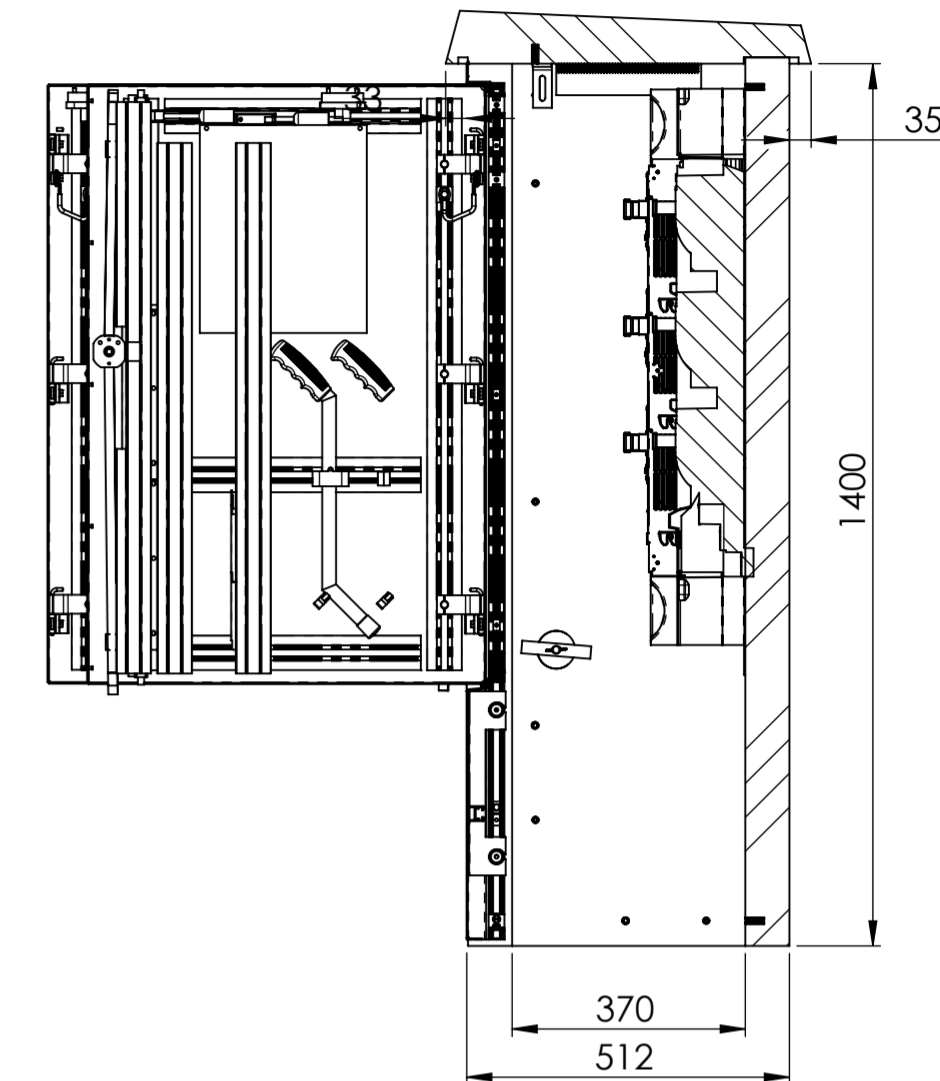
SCHNITT B-B MABSTAB 1 : 12
