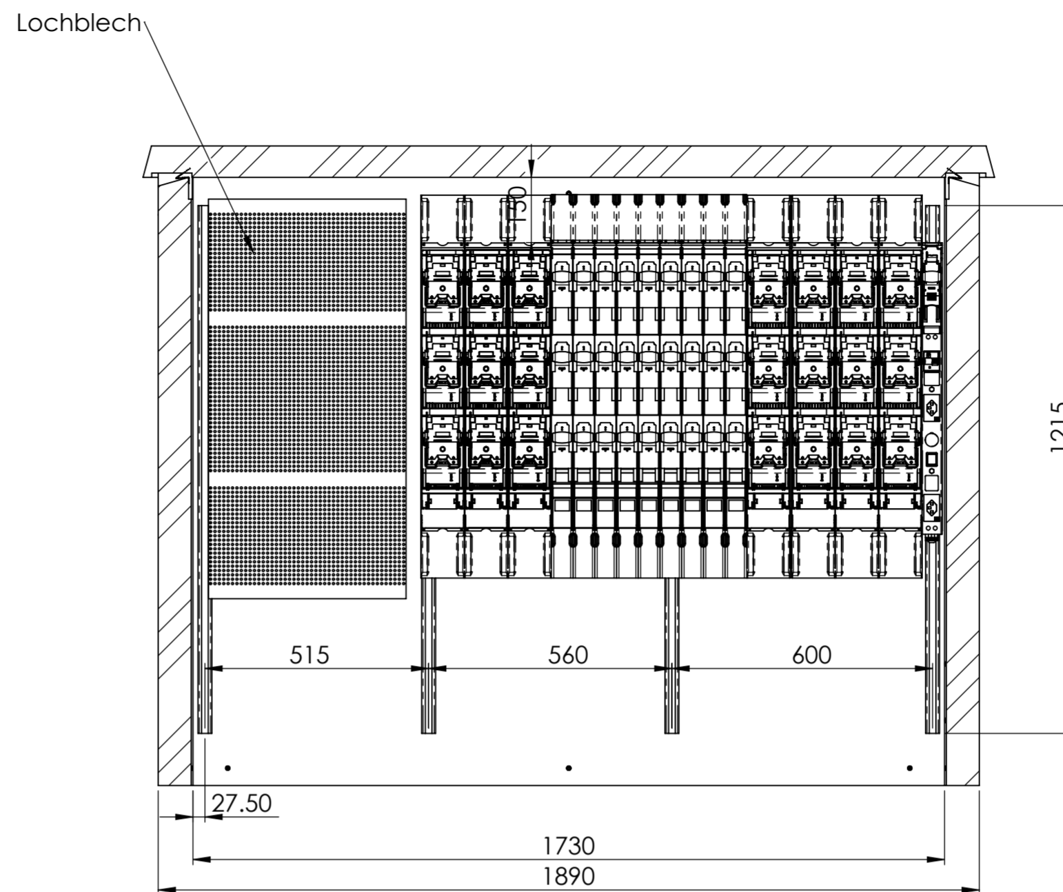
SCHNITT A-A MABSTAB 1 : 12
